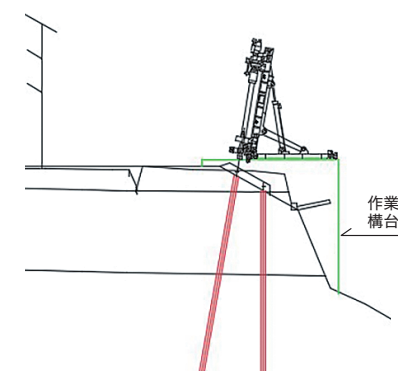
当初計画 スキッド施工図
