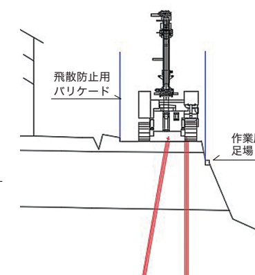
計画変更後 クローラー施工図
